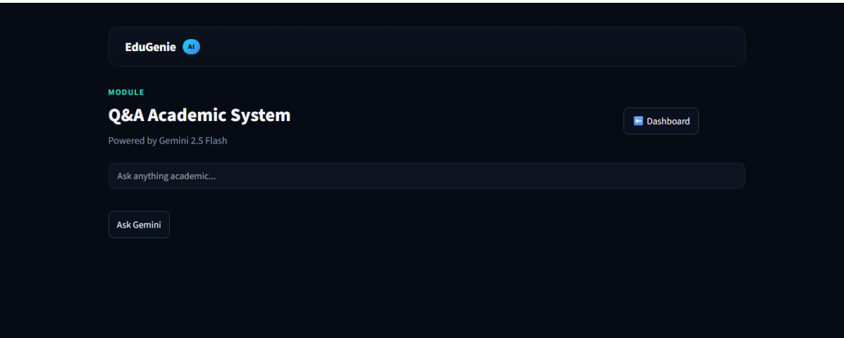
1. Q&A
